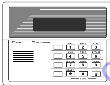
6139 ALPHA KEYPAD
